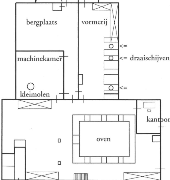
Plattegrond van De Nijverheid, naar een aanvraag hinderwetvergunning van juli 1920. Streekarchief Rijnlands Midden, Alphen a/d Rijn.
