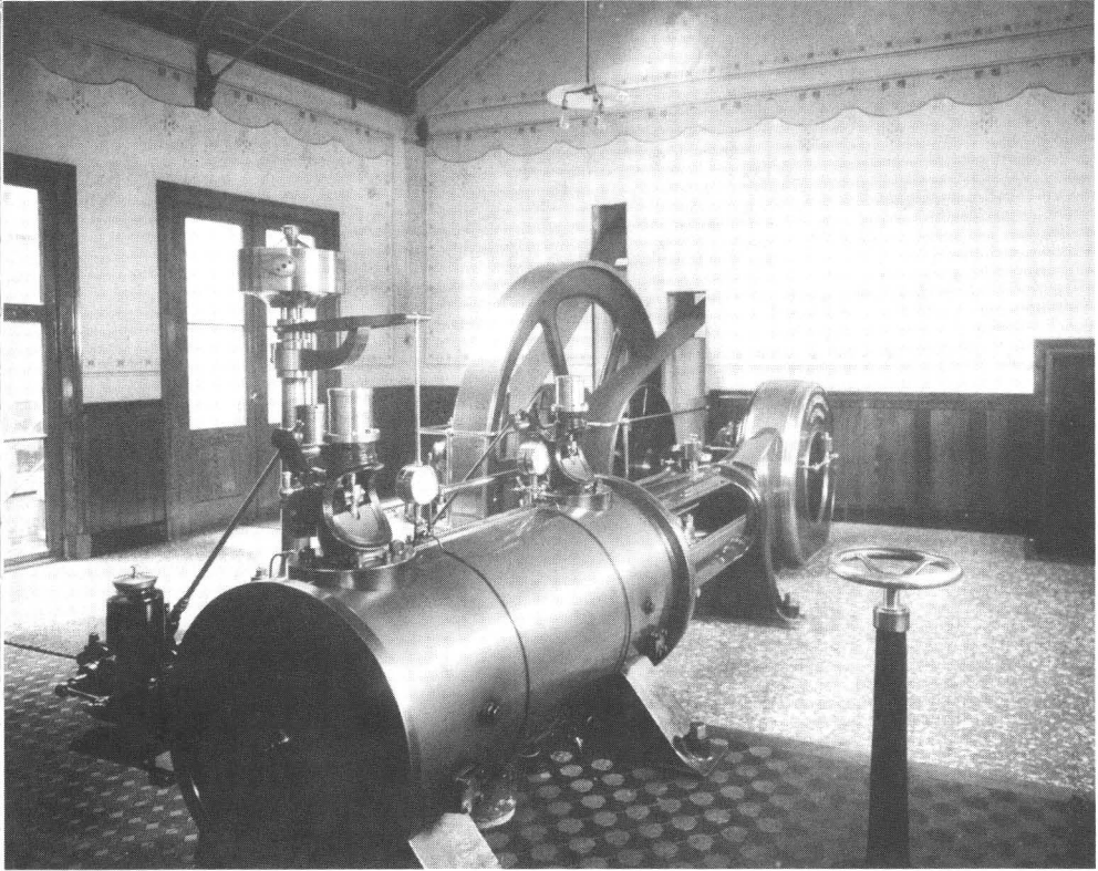
Stoommachine (240 PKg) van de firma Zaalberg, 1913. Foto H. Jonker. GAL, PV 31570, 101.524.
