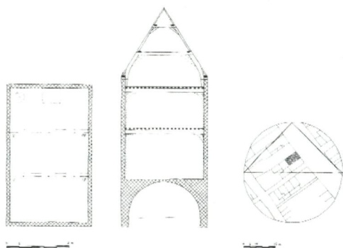
Plattegrond en doorsnede van het voorhuis van Breestraat 95. Tekening Edwin Orsel.
