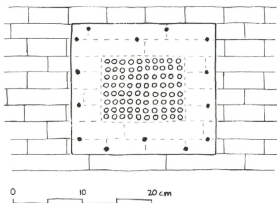
Loden ventilatierooster van de Hartebrugkerk. Tekening Maarten Enderman.
