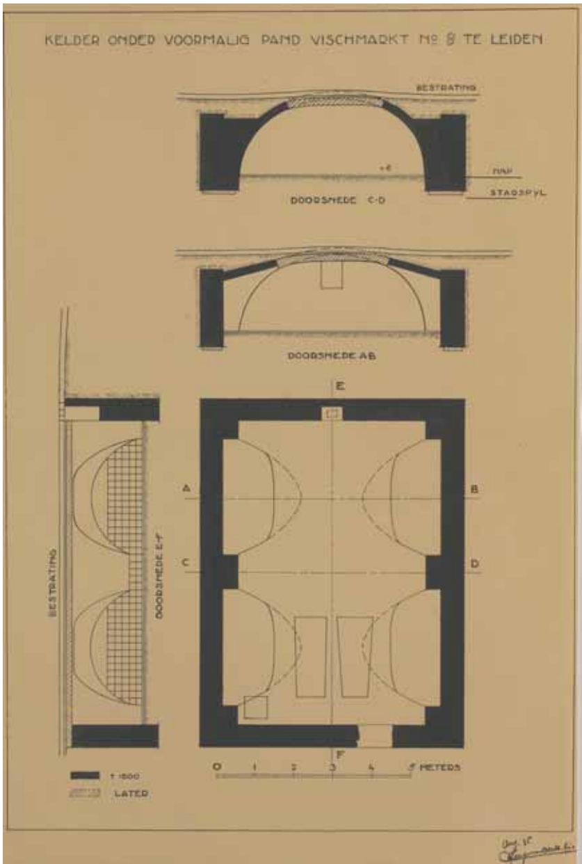
Detail uit een tekening op schaal van de kelder van Vismarkt 9/10, H. van Oerle, augustus 1935, Erfgoed Leiden en Omstreken (PV 16973).
