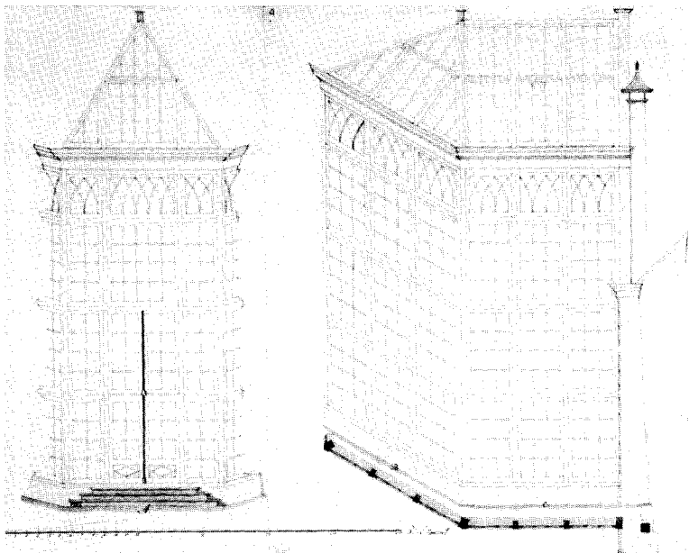
afb. 5b. Als afb. 5a, voor- en zijaanzicht. Niet uitgevoerd ontwerp voor aanbouw aan Oranjerie. Pentekening J. Dobbe, 7818. Leiden, Universiteitsbibliotheek.
