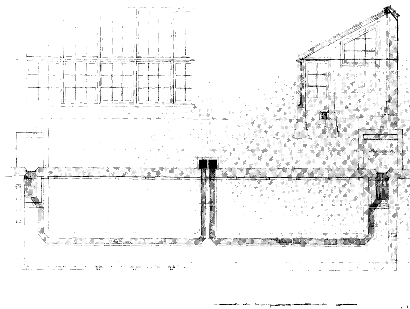
afb. 4. Stookkas, ontwerp. Pentekening J. Dobbe, 1826. Leiden, Universiteitsbibliotheek.
