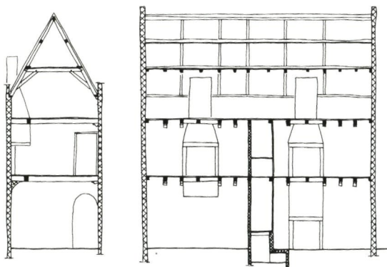
Doorsnedes oorspronkelijke opzet Oude Singel 218 (reconstructie).
