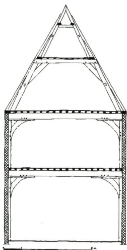
Poging tot reconstructie van de dwarsdoorsnede van het voorhuis van Hogewoerd 33.
