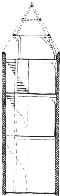
Dwarsdoorsnede van Botermarkt 11.
